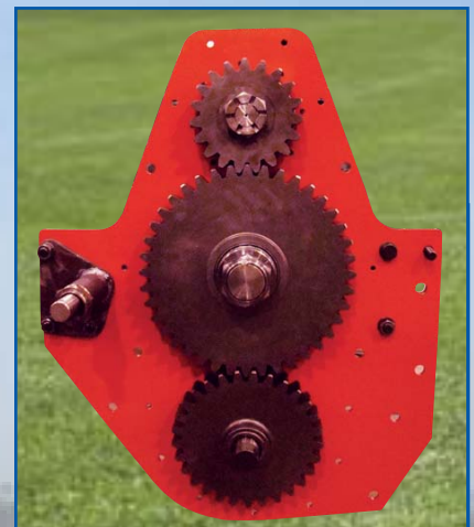
Engranajes laterales Transmission latérale Side drive gears
