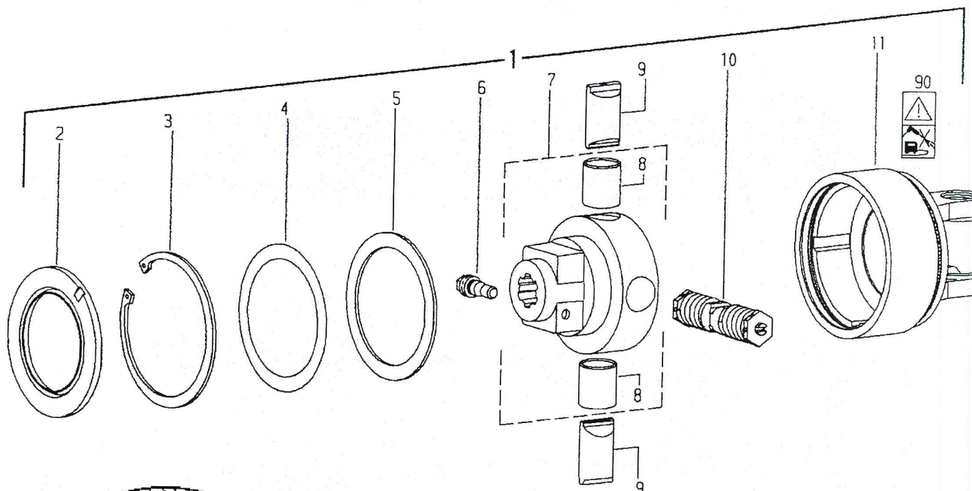
SEZIONE LIMITATORE DESTRO VISTA DAL MOZZO
