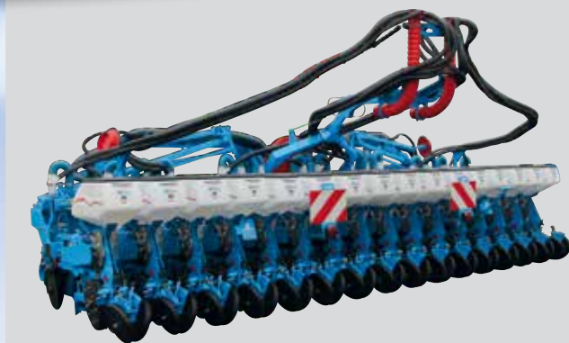
16 rij zaaimachine met een rijafstand op 37,5 cm uitvoering voor gebruik met DUO fronttank
