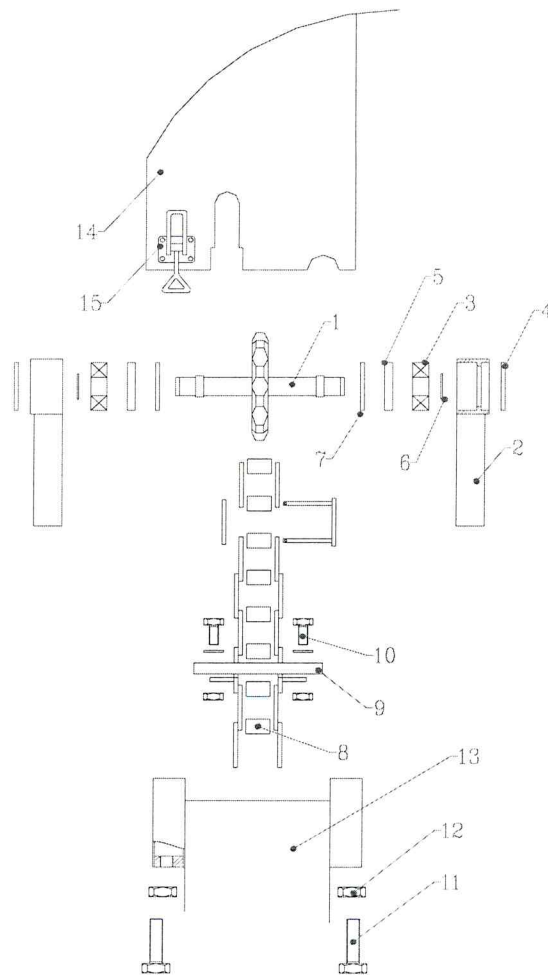
Varaosakuva nro 2 Partspicture No 2 Kiristyspyörä Tightening pulley
