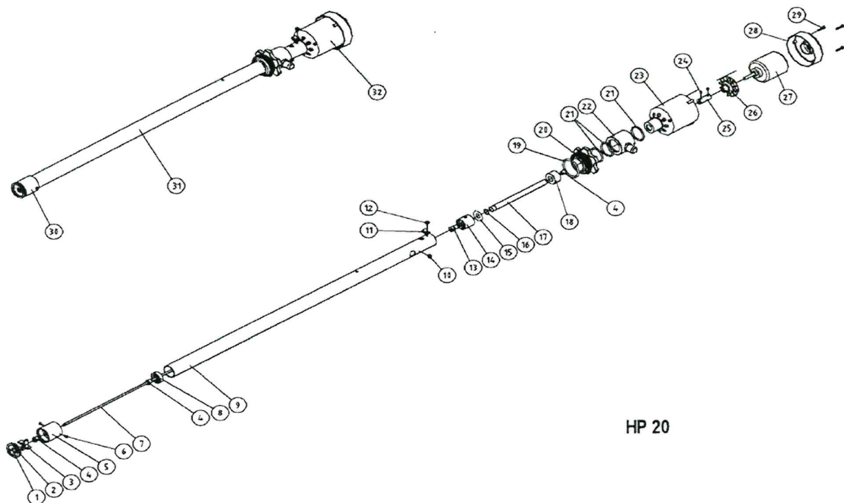
Varaosakuva nro 11 Pumppu
