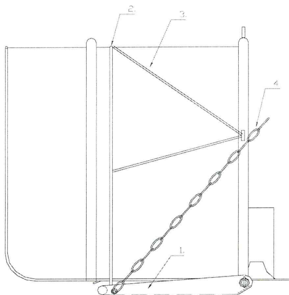
Varaosakuva nro CB 5 CB Painekartio
