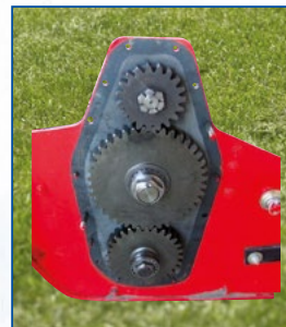
Seitlicher Antrieb Zijdelingse aandrijving
