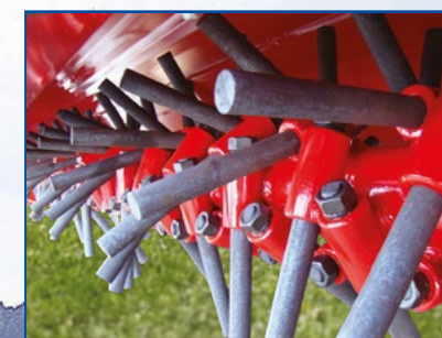
Rotorwelle mit Zinken Rotoras met pennen
