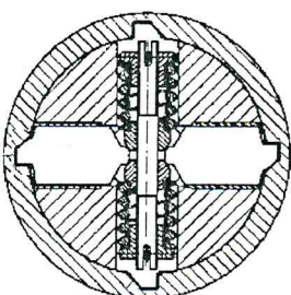
SEZIONE LIMITATORE SINISTRO VISTA DAL MOZZO
