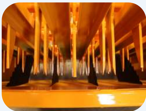
Couteaux fixe sur convoyeur
