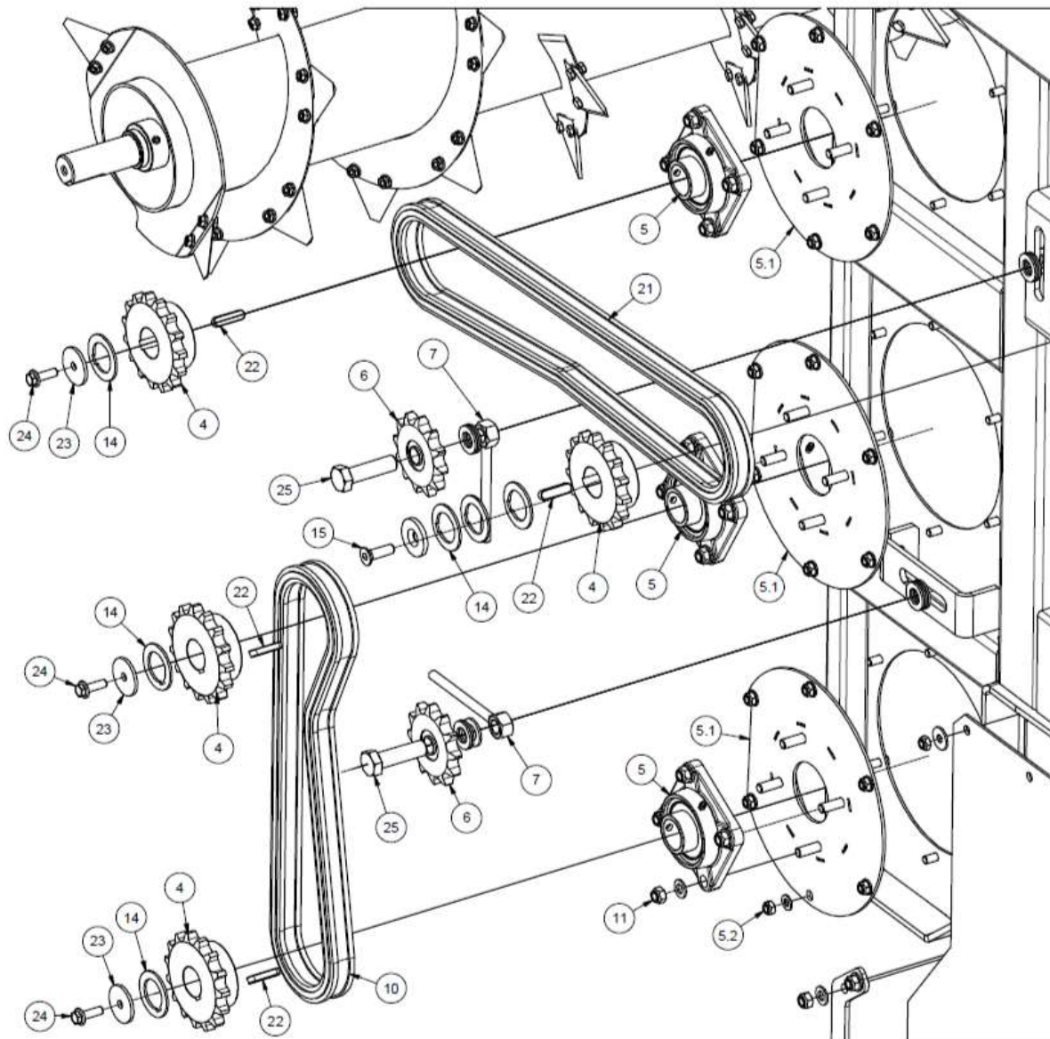
Détail F ( 1 : 5 )
