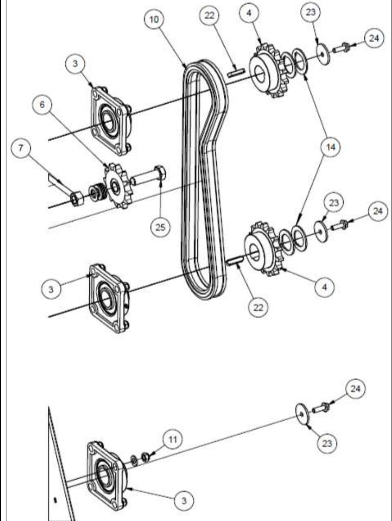
Détail B ( 1 : 6 )
