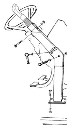
QE-Command bediening - plaatsing van de DIY set in de cabine
