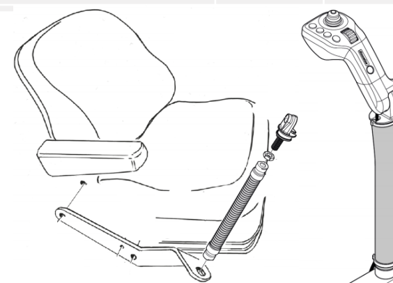
QE-Command bediening - plaatsing van de DIY set in de cabine
