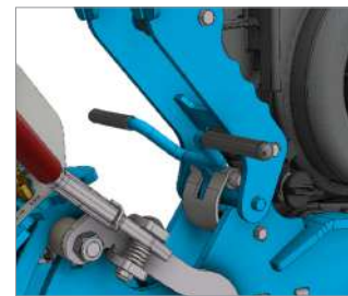
3 VERGRENDINGSSYSTEEM
